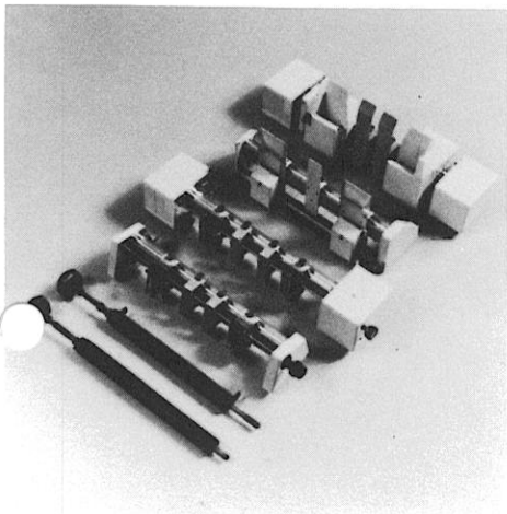
Formularführungen
