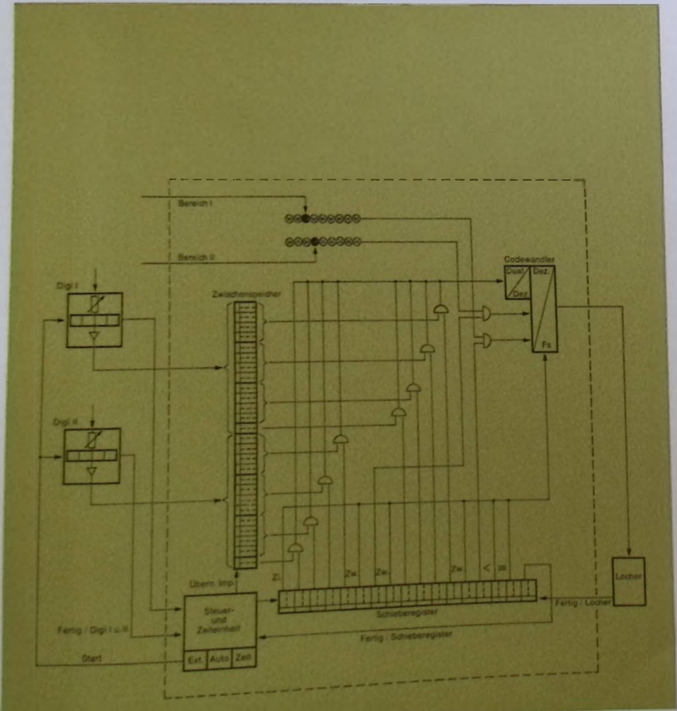
Abb. 4: Vereinfachter logischer Schaltplan.
