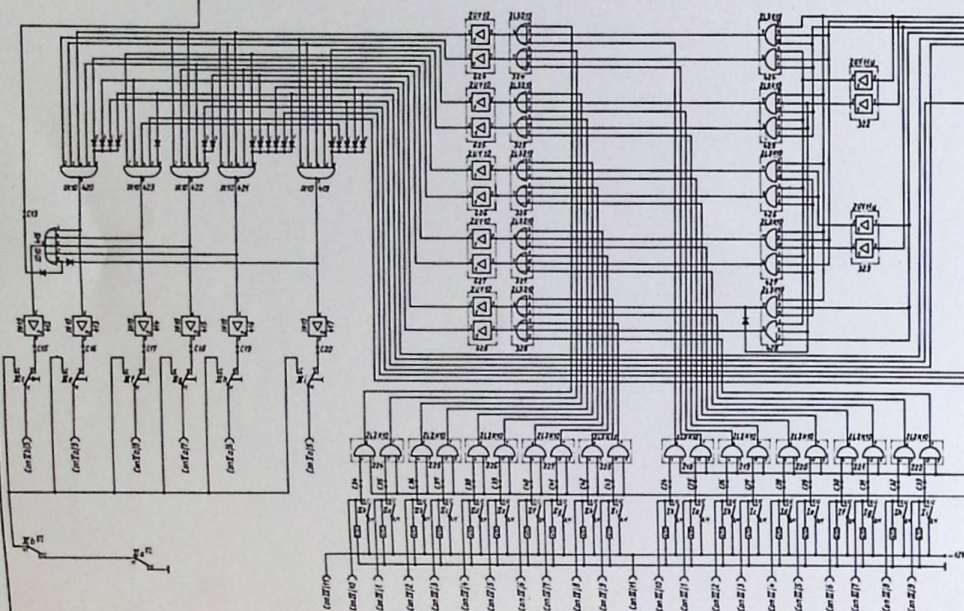
Code-Wandler (Dual-Dez/Dez-FS) mit Leuchterschluss
