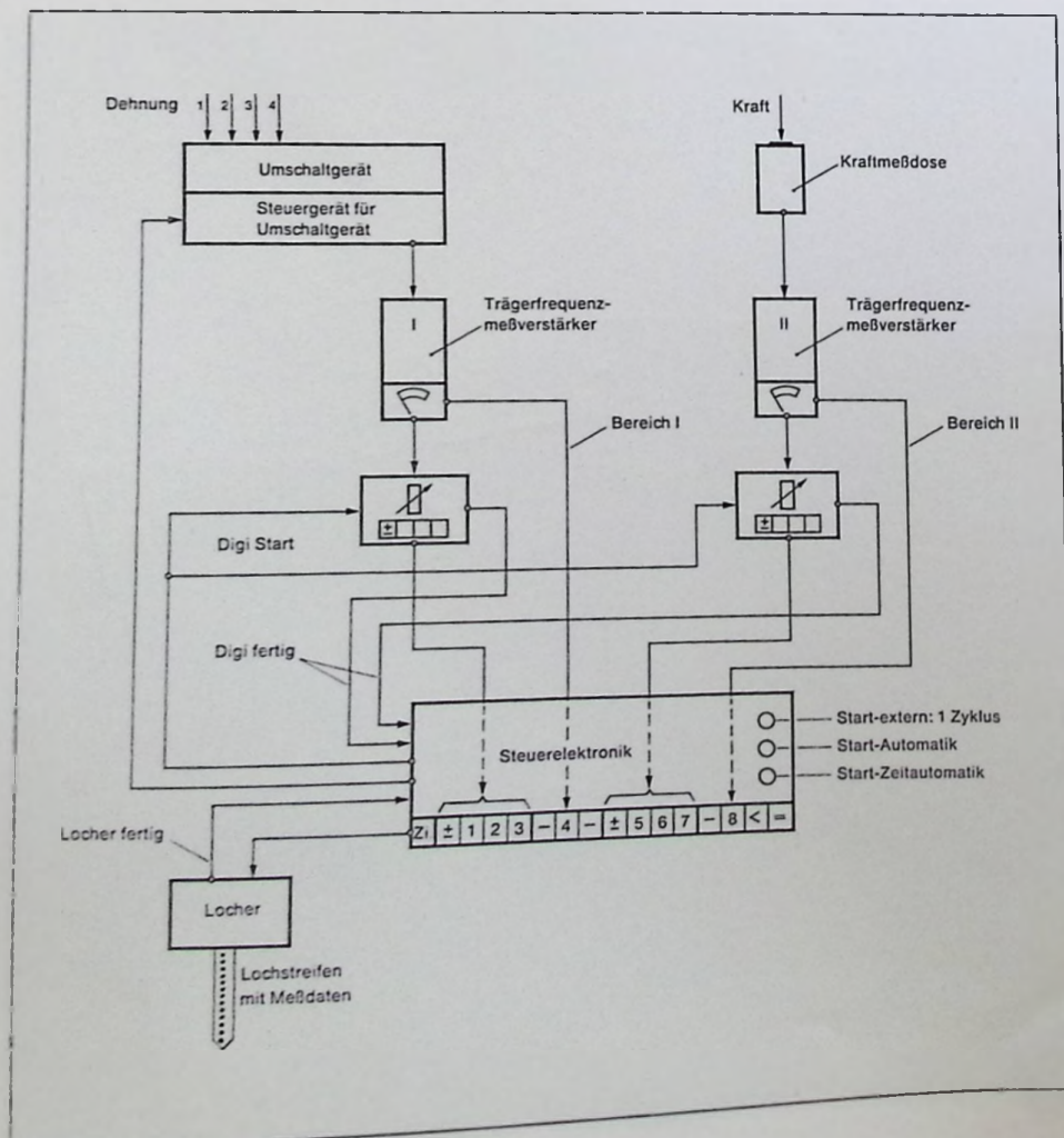
Abb. 1: Blockschaltbild
