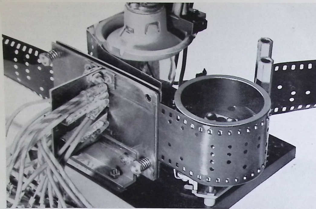
Lichtelektrischer Kinofilm-Lochstreifenstanzer
