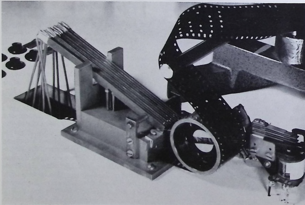
Kinofilm-Lochstreifenstanzer
