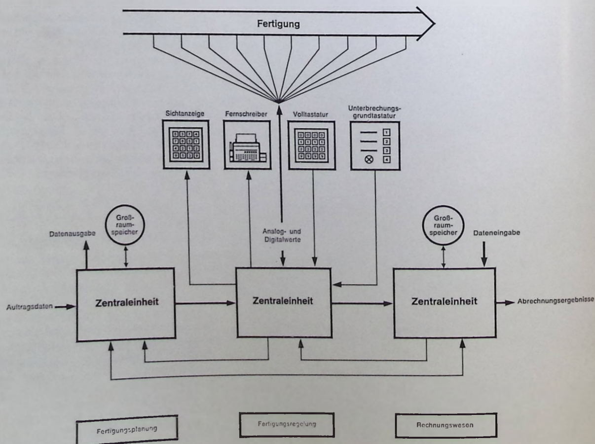
Abb. 8 Informationsfluß: Planung → Fertigung → Rechnungswesen
