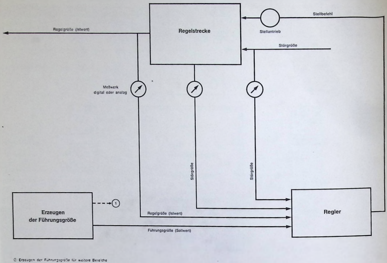
Abb. 2 Regelkreis
