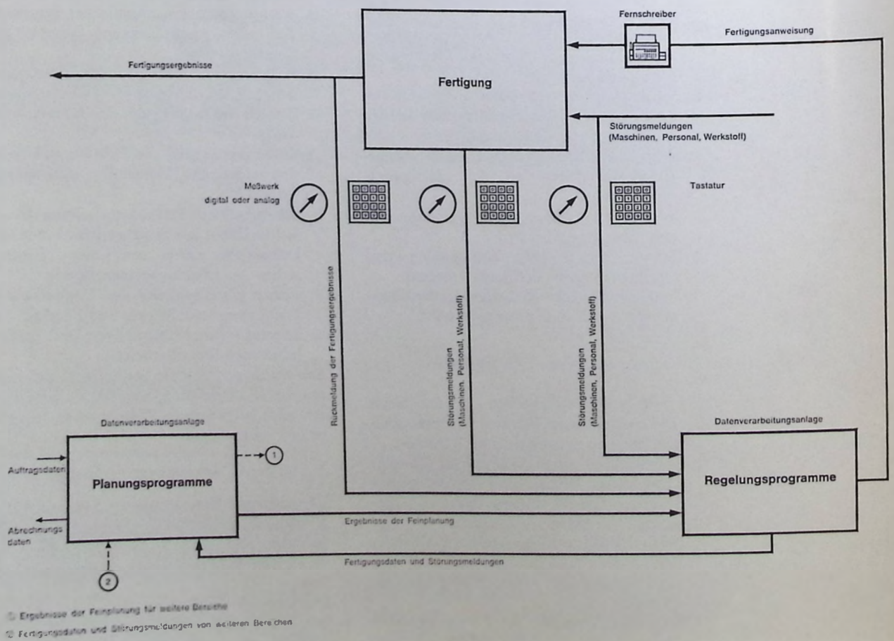
Abb. 3 Fertigungsregelung
