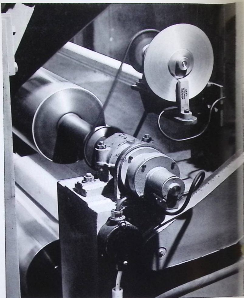
Abb. 13 Geber an einer Fertigungsmaschine: Induktiver Drehzahlgeber zur Ermittlung der Folienlängen (Kettenantrieb), Tachodynamo zur Erzeugung des Produktionskriteriums (auf der Antriebswelle)
