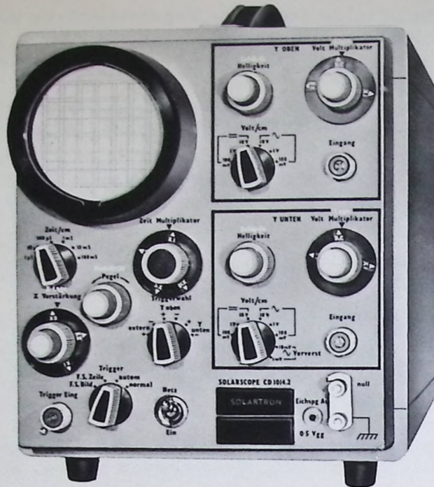
Kathodenstrahloszillograph
