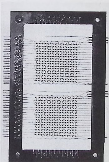
Abb. 3 Kernspeicherebene
