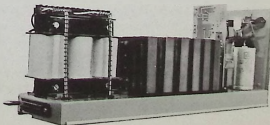
Abb. 6 Netzgerät (von hinten)
