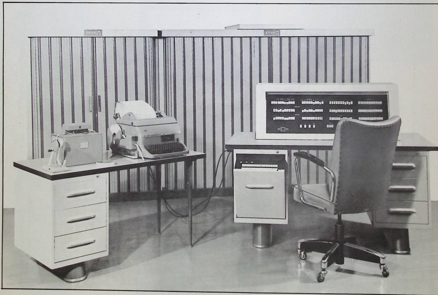
ZUSE Z 23 Gesamtansicht
